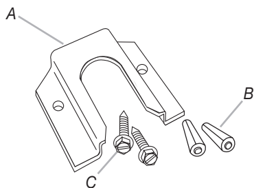
A. Bride antibasculement B. Chevilles en plastique (2) C. Vis à tête Phillips n° 10 x 1/2" (2)
