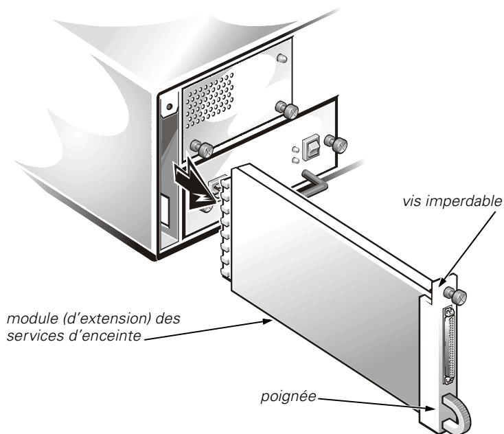
Figure 2-2. Retrait du module existant (côté gauche)
