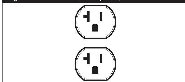
Figura 13 — 120 Volt AC, 20 Amp Receptáculo Doble
