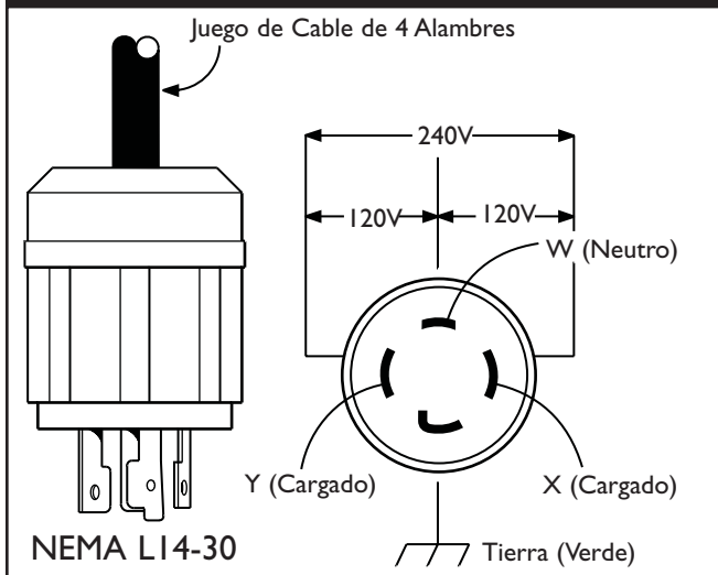
Figura 21 — 120/240 Volt AC, 30 Amp, Receptáculo de Seguridad
