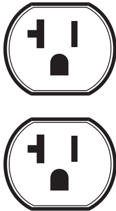
Figura 12 — 120 Voltios AC, 20 Amperios Receptáculo Doble
