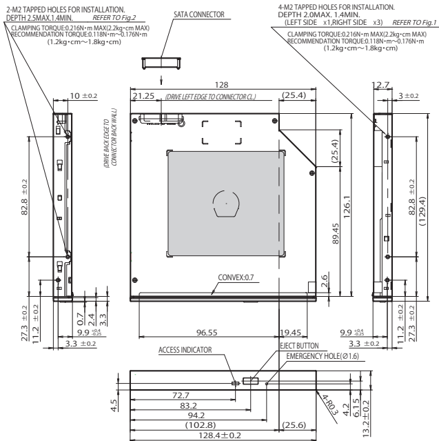
(±0.4) (Unit:mm) DV-28S-W93
