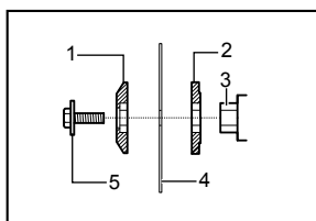
1. Bague externe 2. Bague interne 3. Axe 4. Lame 5. Boulon hexagonal
