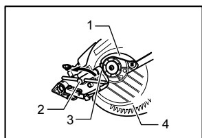
1. Couvercle central 2. Clé à douille 3. Boulon hexagonal 4. Capot de sécurité
