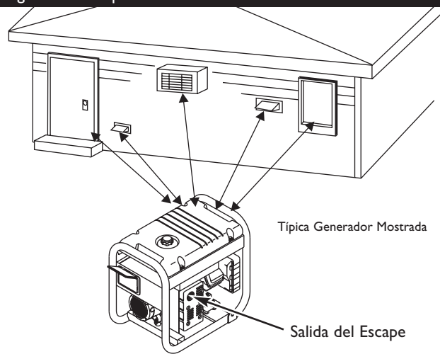
Figura 13 — Espacio Libre Alrededor del Generador
