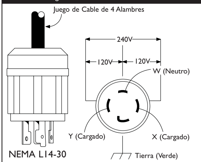
Figura 15 — 120/240 Volt AC, 30 Amp, Receptáculo de Seguridad
