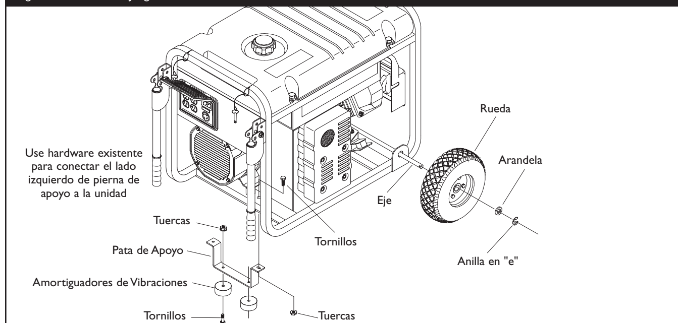
Figura 11 — Instale el Juego de Ruedas
