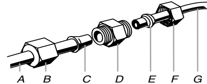
A. Tubería de agua al refrigerador B. Tuerca (provista) C. Bulbo D. Acoplamiento (adquirido) E. Férula (adquirida) F. Tuerca (adquirida) G. Línea de agua de la casa
