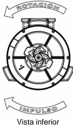
Fig. A – Rotación correcta del rotor, modelos trifásicos
