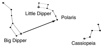
Fig. 52: Locating Polaris.
