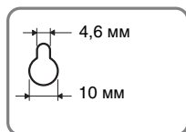
Отверстие в задней панели динамика
