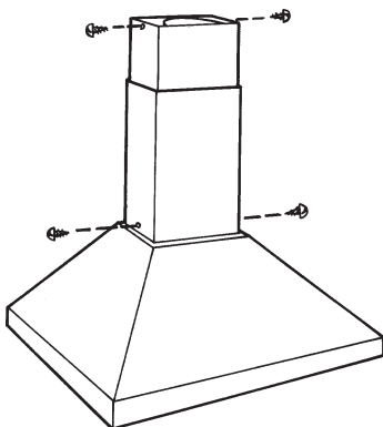
FIXEZ LE TUYAU À LA HOTTE ET A L'ÉTRIER AU MOYEN DES VIS D'ASSEMBLAGE (3,9x9,5mm)
