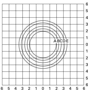
ACN15S5C.IES 150-Watt HPS 16,000-Lumen Clear ED-23.5 Lamp Type V Cutoff
