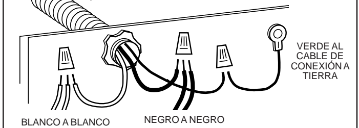
FIG. 2 Todas las conexiones eléctricas se deben hacer de acuerdo con las ordenanzas del código local. Si no está familiarizado con los procedimientos de cableado eléctrico, procure los servicios de un electricista calificado.
