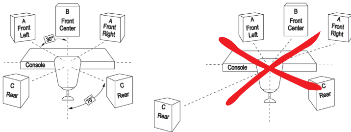
Abbildung 4: Surround-Anordnung
