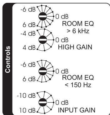
Abbildung 6: Kontrollpanel P33A
