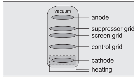
Fig. 4.6: Pentode
