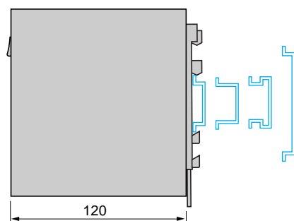
ASI ABLB300●
