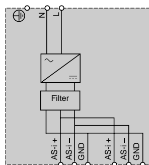
ASI ABLB300●
