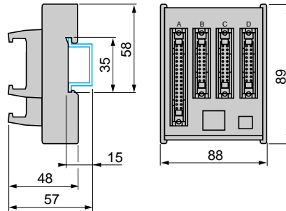
ABE-7ACC03
