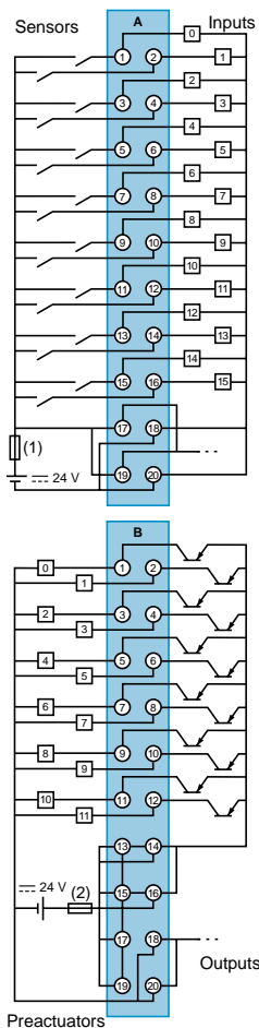
TSX DEZ 28DTK
