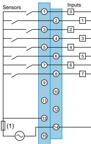
TSX DEZ 08A4/08A5
