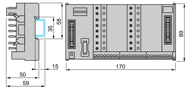
ABE-7TES160
