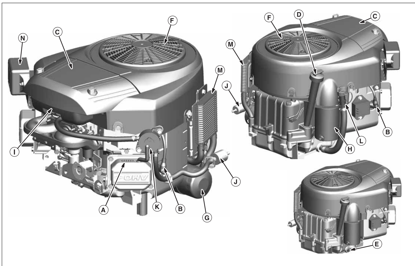
Motorens betjeningsanordninger
