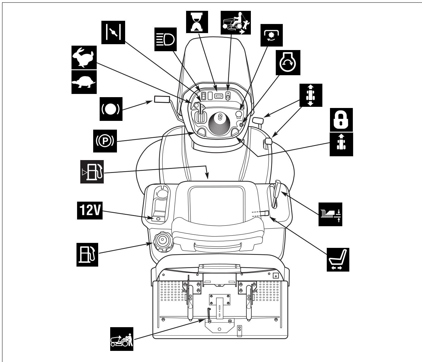
Traktorkontroller
