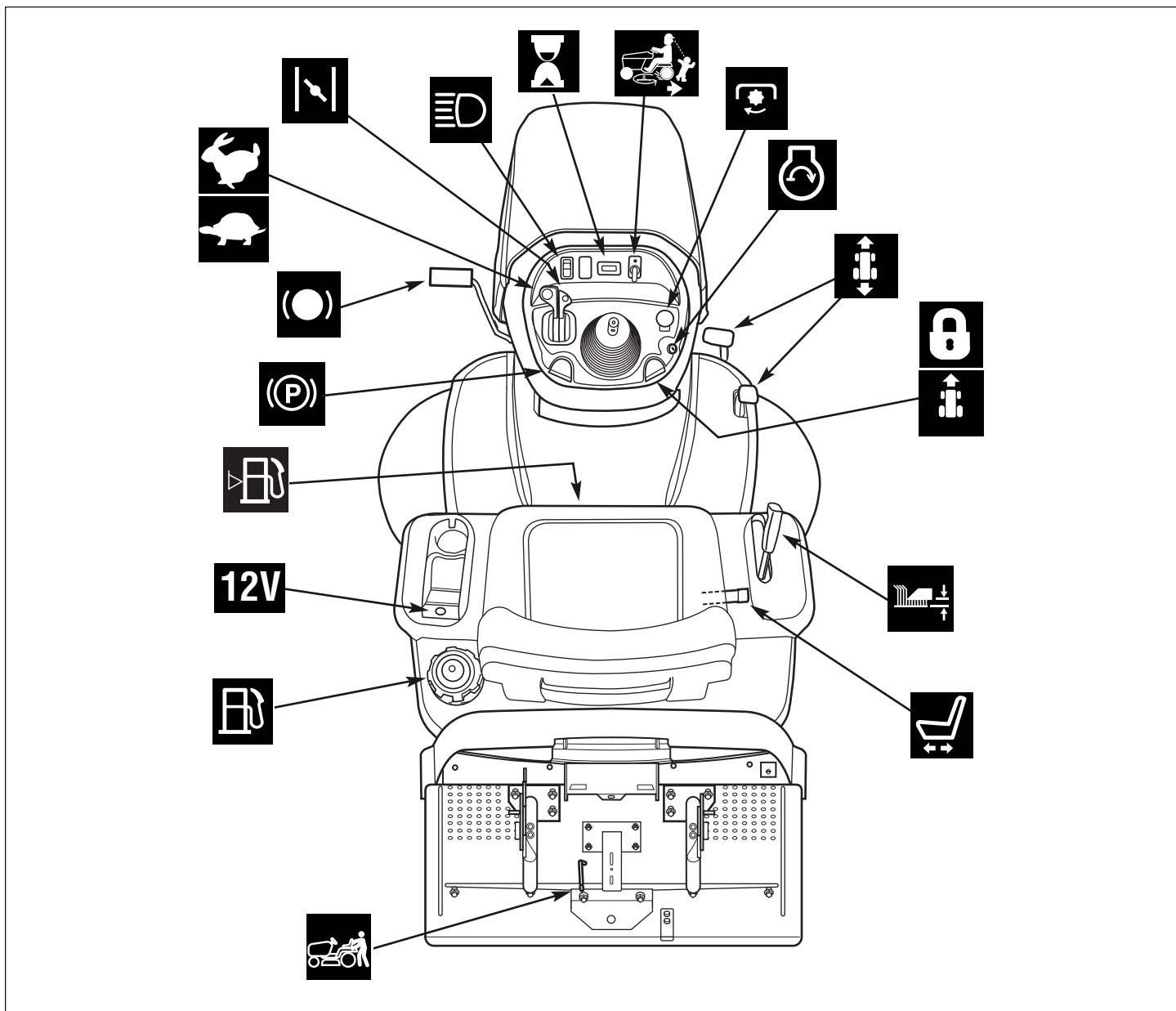
Bedieningselementen van de zitmaaier
