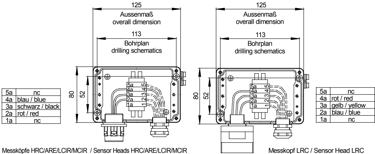
Bild 1 / Picture 1: Messköpfe für brennbare Gase / Sensor heads for combustibile gases
