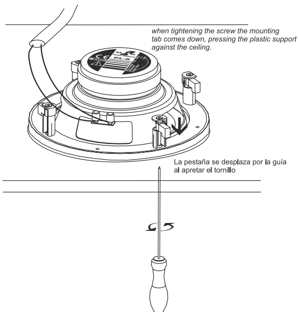
Figura 10 – funcionamiento del sistema de fijación: al apretar el tornillo la pestaña se desplaza hacia abajo oprimiendo el soporte de plástico contra el techo.
