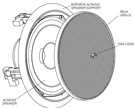
Figura 1 – vista delantera CL-5
