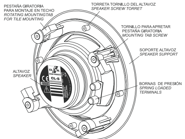
Figura 2 – vista trasera CL-5
