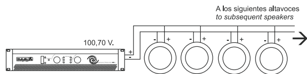
Figura 5 - Conexión en paralelo de unidades con transformador
