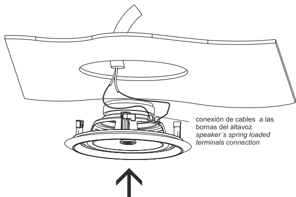
Figura 8 – conexión de terminales; posicionamiento del altavoz
