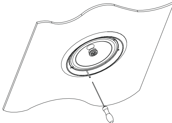
Figura 9 – fijación del altavoz al techo
