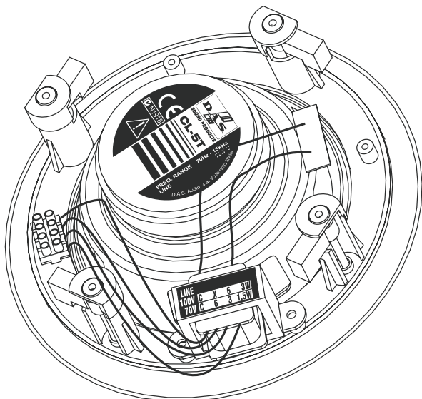
Figura 7 – CL-5T; terminales para selección de potencia
