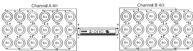
Figura 4.1 – conexión serie-paralelo con mayor número de unidades por canal
