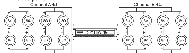
Figura 4 - conexión serie-paralelo
