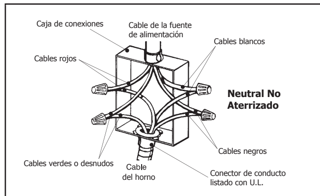
Figura 4: Conexión con cuatro hilos
