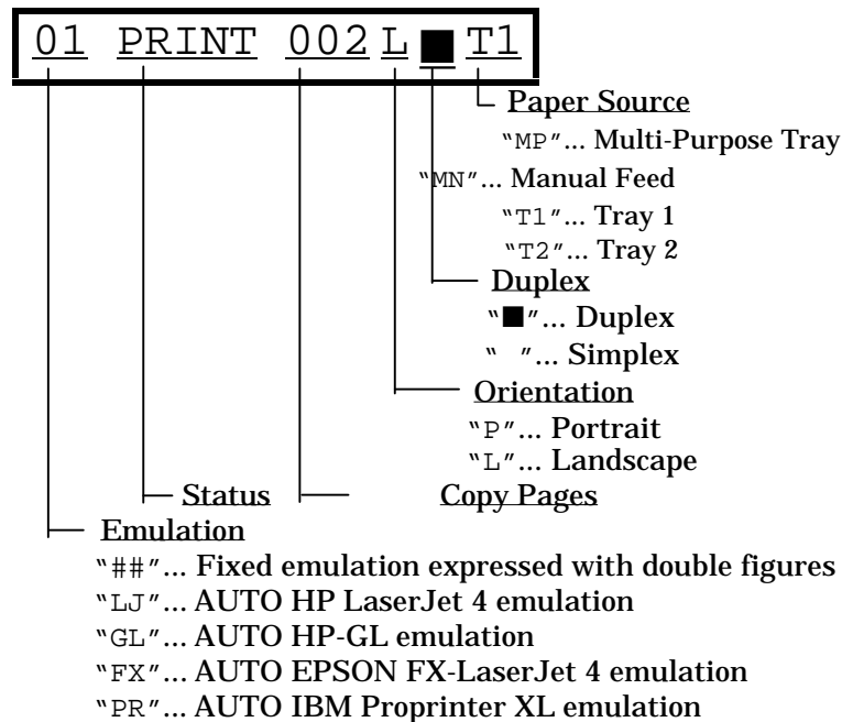
Fig. 4-2 Display
