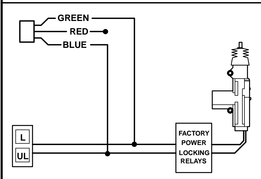
NEGATIVE TRIGGER DOORLOCK WIRING
