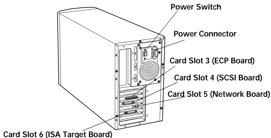
Figure 1-11. CS-6000N Back
