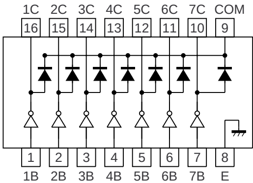
IC8: VHiULN2003AN/ (ULN2003ANS)
