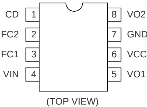
IC6: VHiNJM2113M-1 (NJM2113M)
