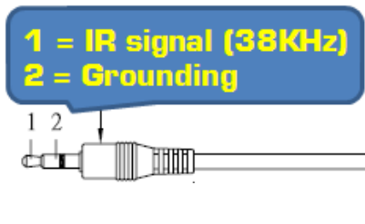
IR Blaster
