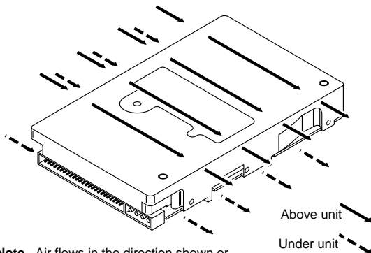
Figure 4. Suggested air flow Abbildung 4. Empfohlener Luftstromverlauf
