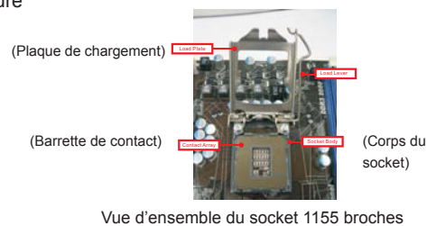
Vue d'ensemble du socket 1155 broches
