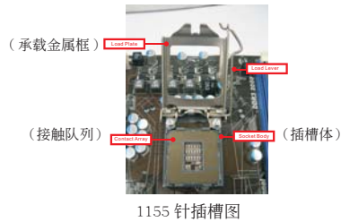
1155 针插槽图
