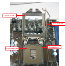
1155 ピンソケットの概要
