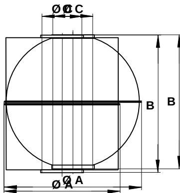
Form Z - Zylinderschwimmer Form K - Kugelschwimmer
