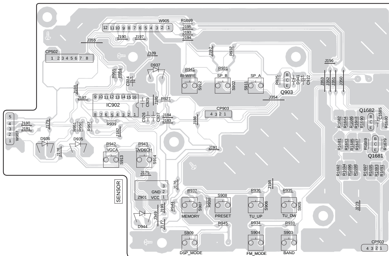
G KEY P.C.B. (REP3020A-S)
