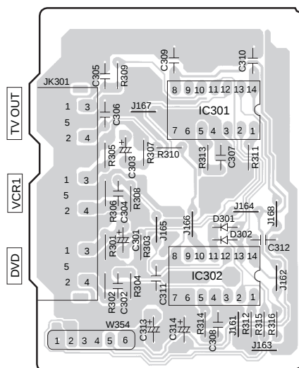
F S-VIDEO P.C.B. (REP3020A-S)
