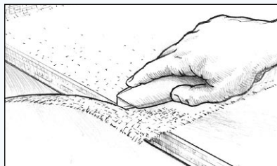
Slika 25 Višak platna odstraniti skalpelom poslije gel faze ,ali prije potpunog otvrdnjavanja
