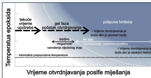
Figure 1 Prilikom otvrdnjavanja epoksid prolazi kroz tri faze: tekuću, gel, tvrdnu
