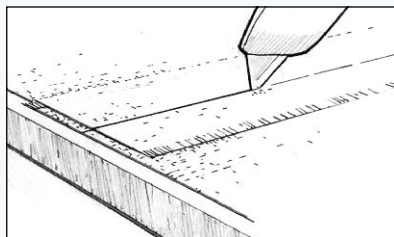
Slika 26 Odvojiti preklepe platna poslije gel faze
