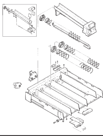
Snack Shelf 5.17
