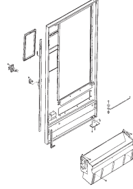
Door - Inside Front Odyssey 5.05
