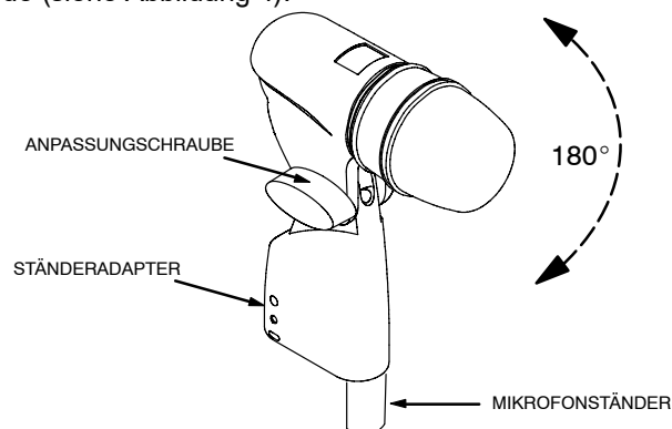
EINGEBAUTER STATIVADAPTER FÜR BETA 56A ABBILDUNG 4
