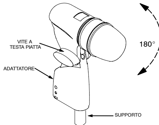
ADATTATORE INCORPORATO PER SUPPORTO BETA 56A FIGURA 4
