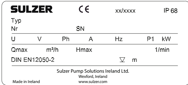
Abb. 1: Typenschild
