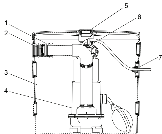
Abb. 3: Sanimax MF
