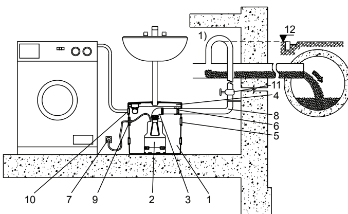
Abb. 5: Installationsbeispiel
