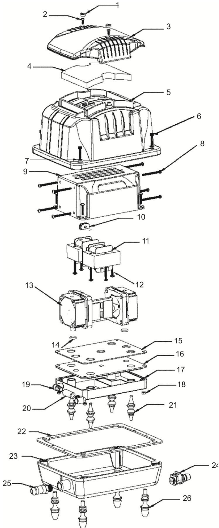
AirTec 600 – 1200 – 2400
