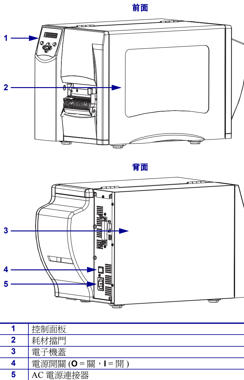
圖 2 • 外部 印表機
