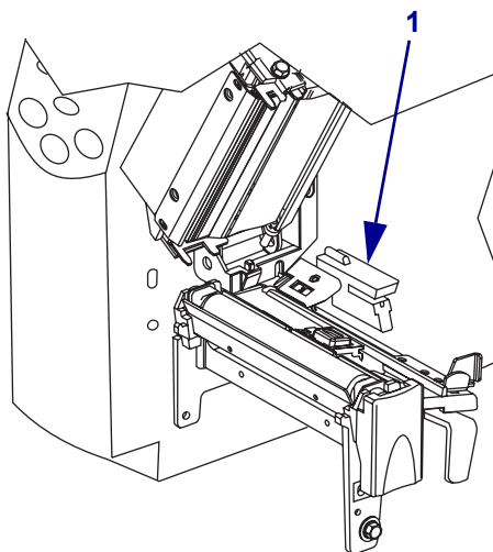
圖 21 • 傳輸感應器
