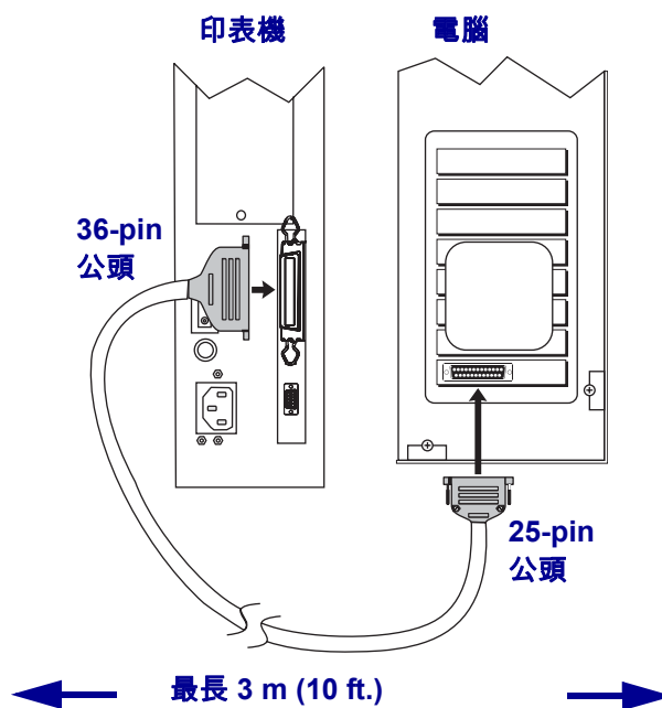
圖 8 • 使用平行埠通訊
