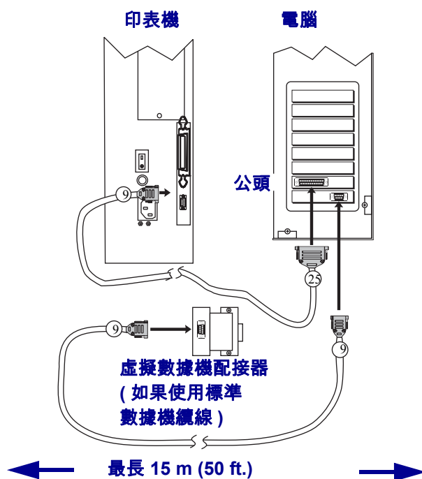
圖 7 • 使用序列資料埠通訊
