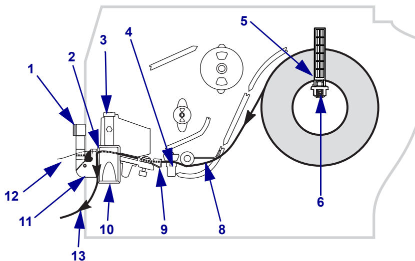
圖 18 • 剝離模式
