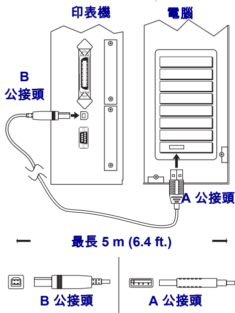
圖 9 • 使用 USB 埠通訊
