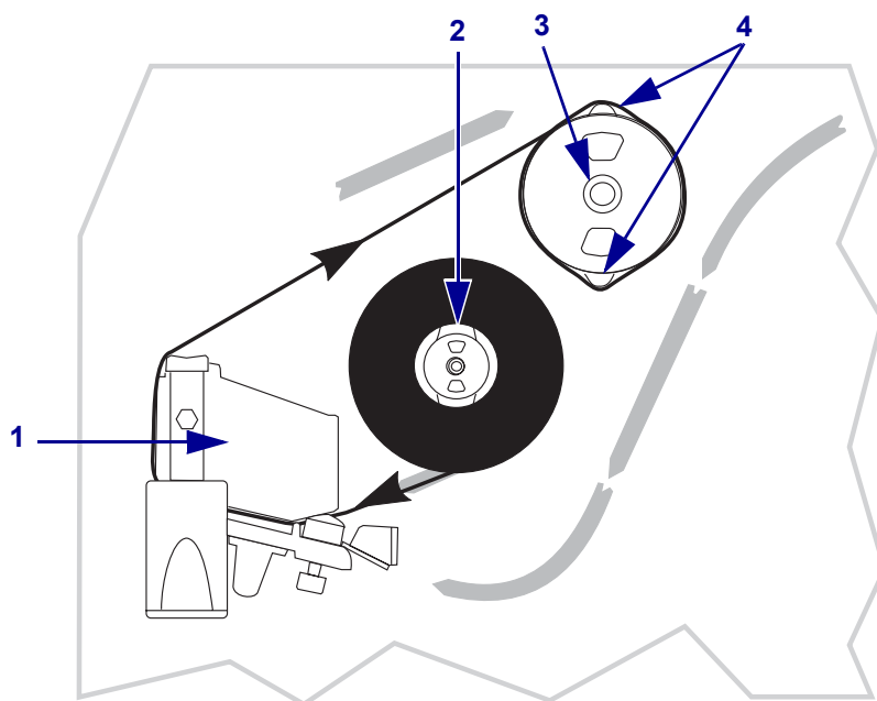
圖 19 • 色帶路徑
