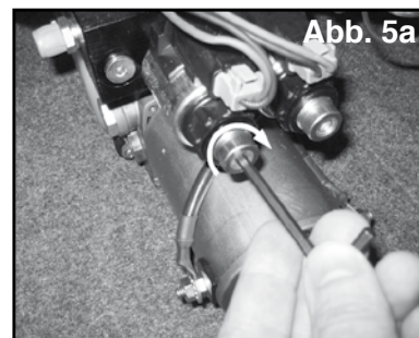
Abb. 5a Tourner dans le sens des aiguilles d'une montre pour ouvrir la valve
