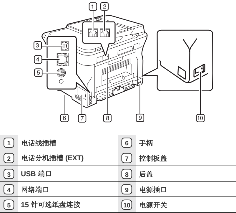
后视图
