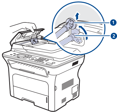
1 套管 2 ADF 滚筒
