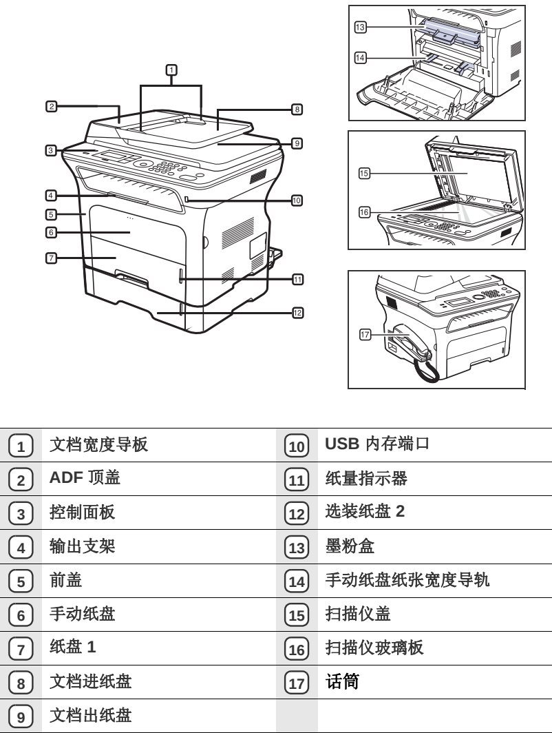
前视图
