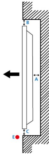
<侧面视图>
