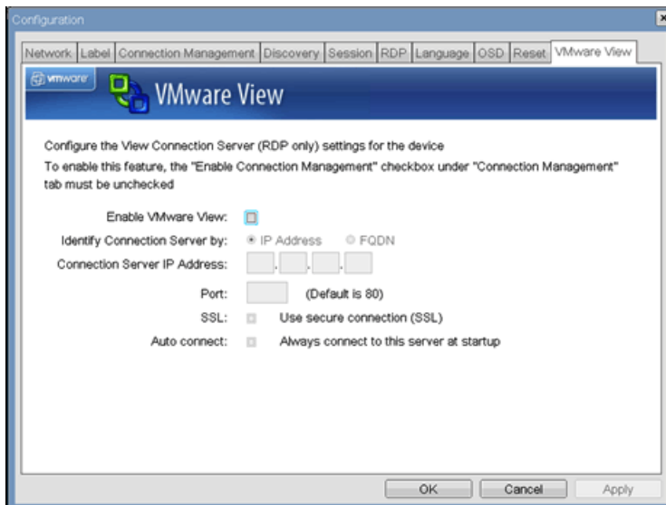
Abbildung 2-11: Konfigurieren von <VMware View>
