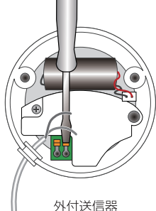
外付送信器
