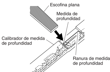
Figura 24 - Calibrador de medida de profundidad en la cadena
