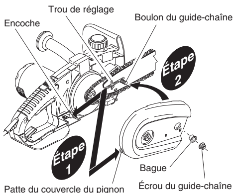
Figure 7 - Installation du couvercle du pignon
