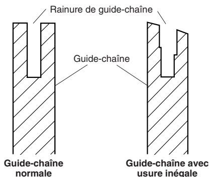
Figure 19 - Coupe transversale d'une guide-chaîne montrant une usure inégale
