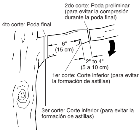
Figura 19 - Poda de una rama
