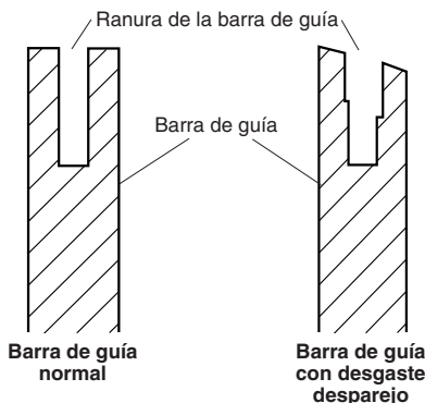
Figura 20 - Sección transversal de la barra de guía que ilustra el desgaste desigual de la misma
