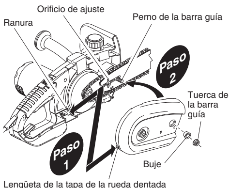
Figura 7 - Instalación de la tapa de la rueda dentada
