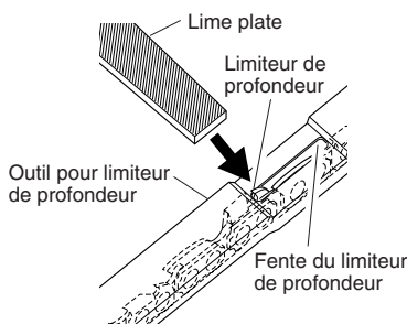
Figure 23 - Position de l'outil pour limiteur de profondeur sur la chaîne
