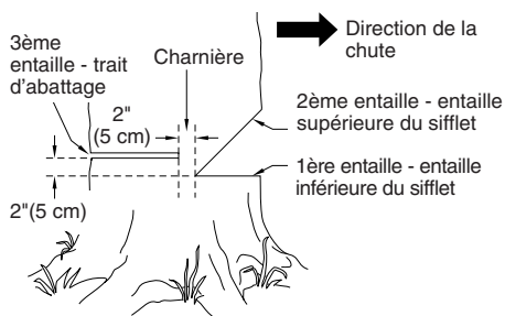
Figure 13 - Abattage d'un arbre
