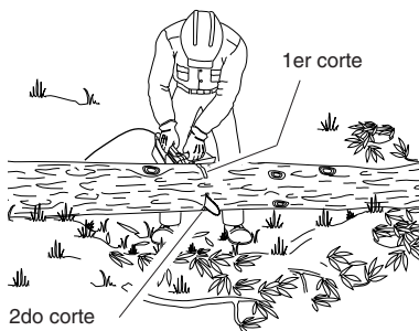
Figura 18 - Trozado del tronco apoyado sobre ambos extremos
