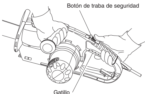
Figura 12 - Posición del gatillo y de la traba de seguridad
