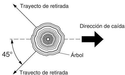
Figura 13 - Trayecto de retirada de un árbol
