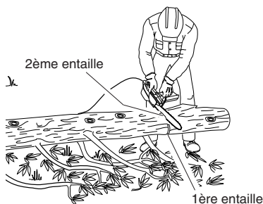
Figure 16 - Tronçonnage d'une bille soutenue à une extrémité
