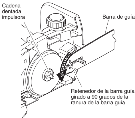
Figura 5 - Bloqueo del retenedor de la barra guía
