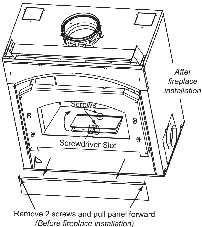
Figure 30-A Accessing Fan Motor
