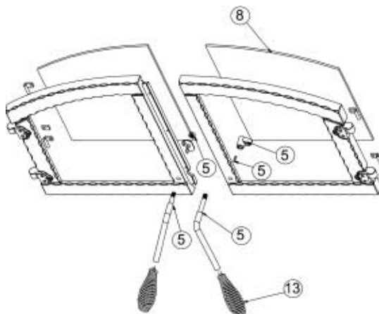
Door Assembly
