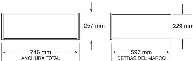
Medidas totales: frente de cajón integrado
