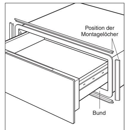
Einfassung der Wärmeschublade installieren
