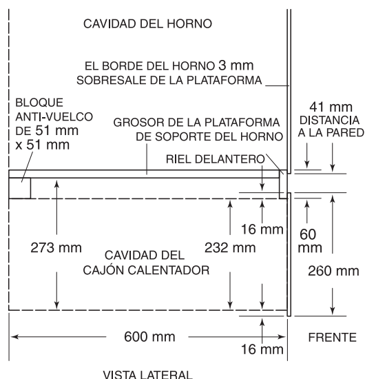
Instalación con horno incorporado: frente de cajón de acero inoxidable
