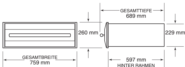
Gesamtabmessungen – Schubladenfront aus Edelstahl
