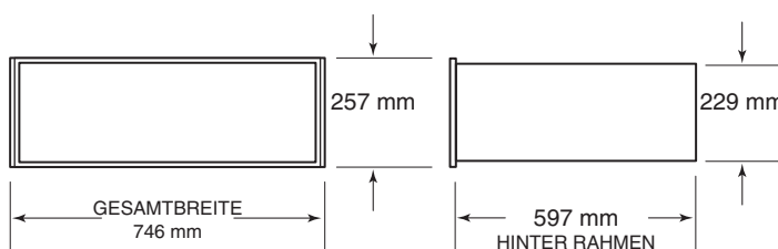
Gesamtabmessungen – Integrierte Schubladenfront
