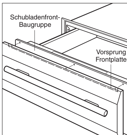
Griff anbringen
