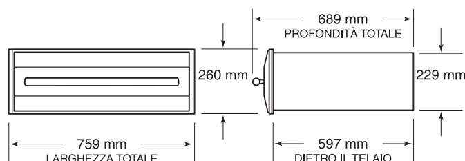
Dimensioni generali - Mascherina anteriore in acciaio inossidabile
