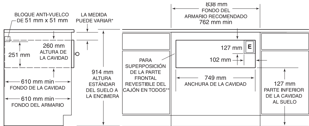
Medidas totales: frente de cajón integrado
