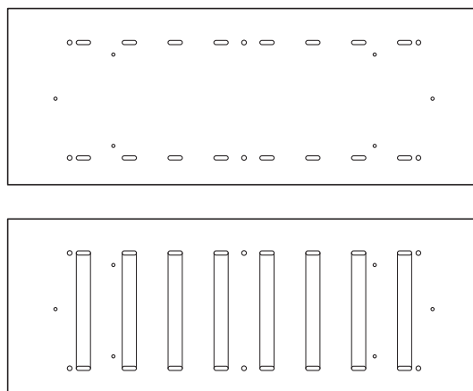
Rückansicht der Dekorplatte
