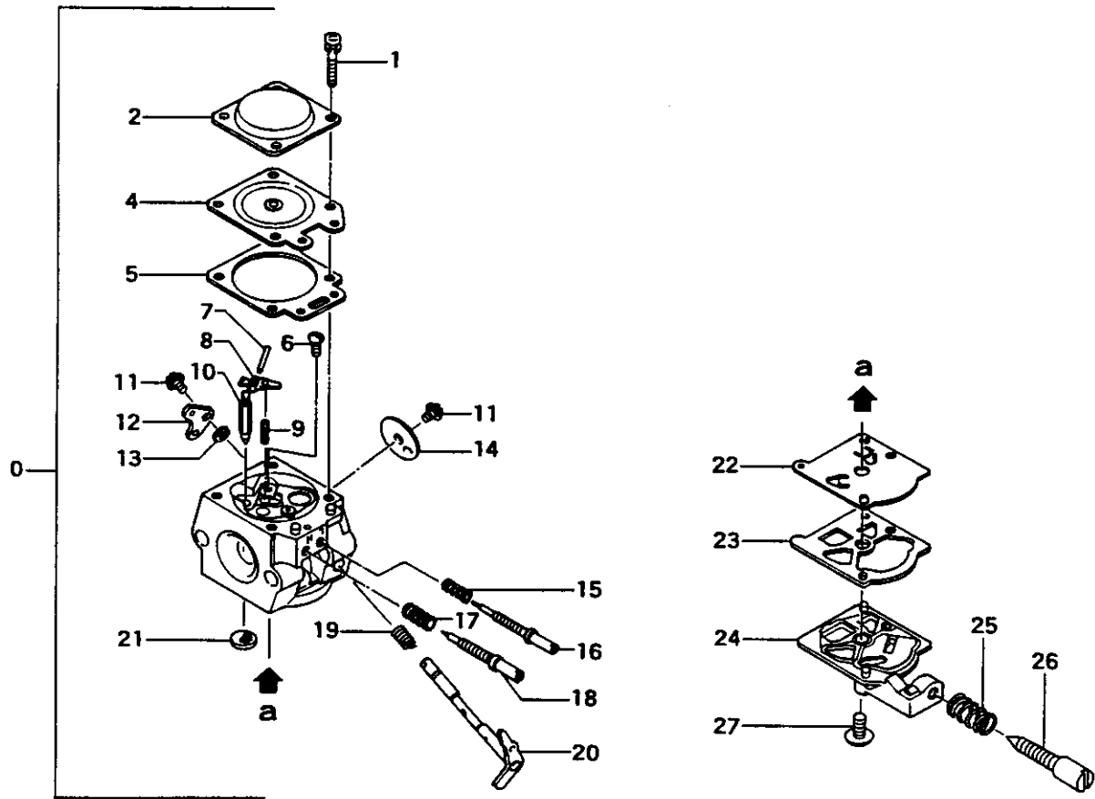
FIG.5 CARBURETOR
