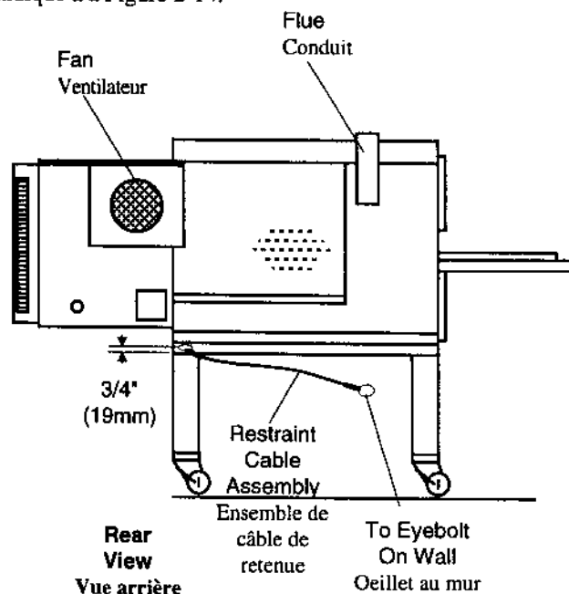
Figure 2-12. Single Oven Flue Installation Figure 2-12. Installation du conduit d'évacuation pour four unique
