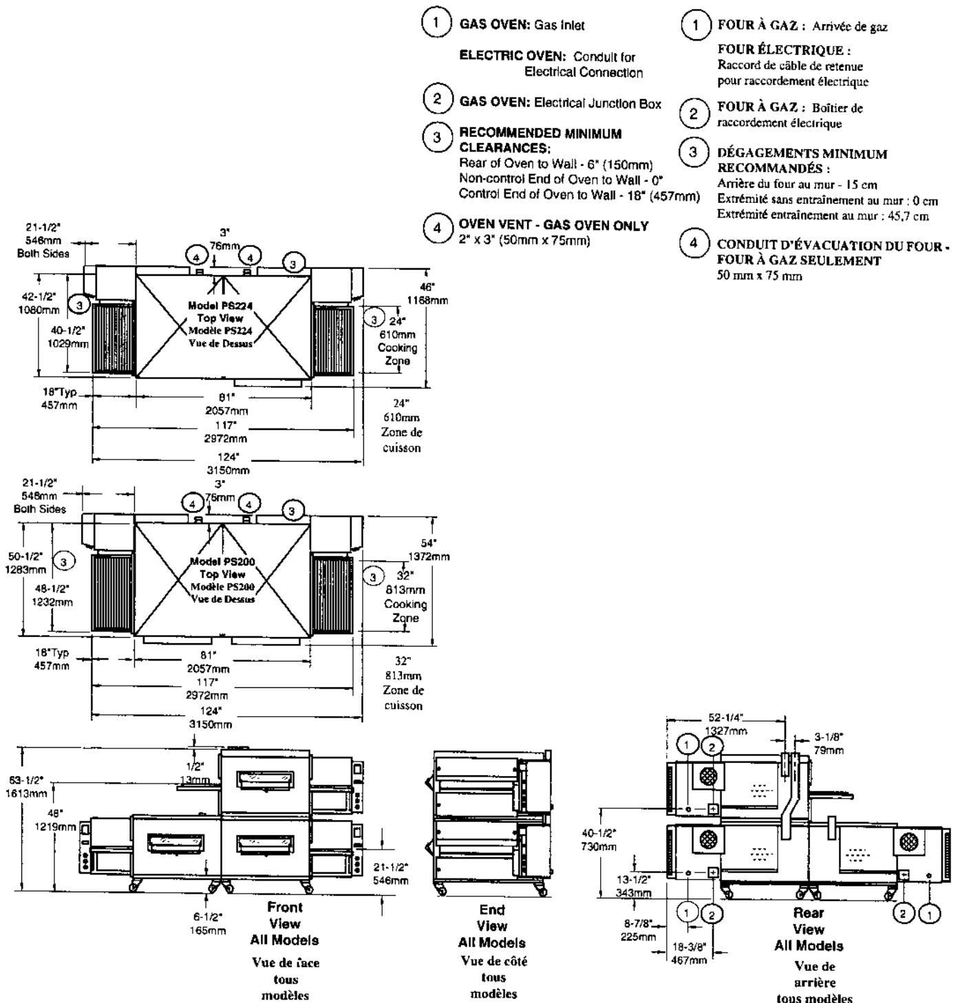
Figure 2-10. MODÈLES PS200 & PS224 FOURS TANDEMS MODÈLES PS200 ET PS 224 AVEC UN FOUR SUPERPOSÉ - DIMENSIONS
