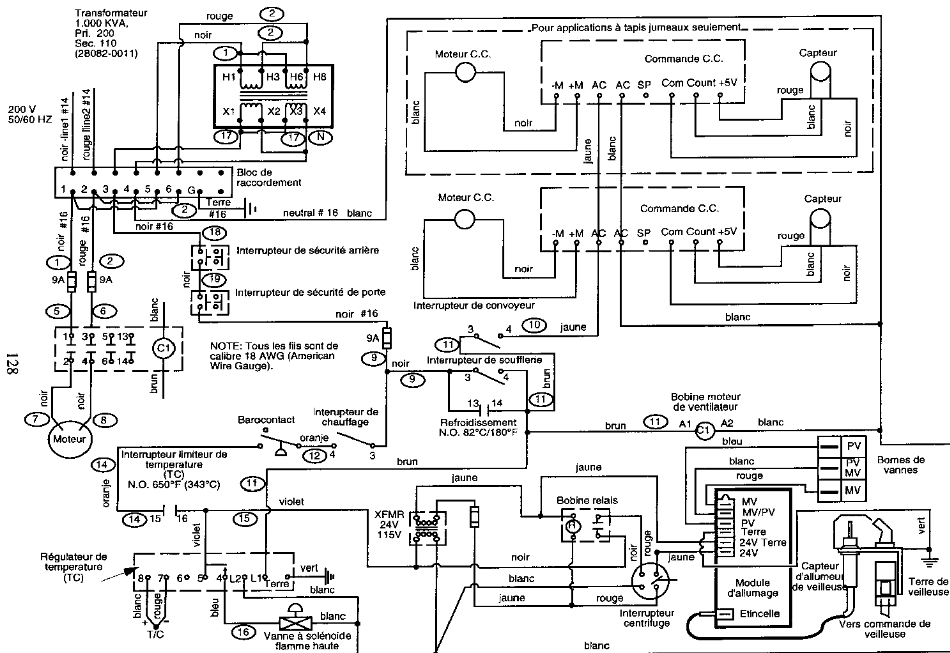
SCHEMA DE CÂBLAGE DU FOUR À GAZ SÉRIE PS200 Moteur de soufflerie 200 V, 50/60Hz, 4., 1 A, bipolaire, 3 fils (2 conducteurs, 1 terre), monophasé, Circuit de commande 120V, EXPORTATION SEULEMENT
