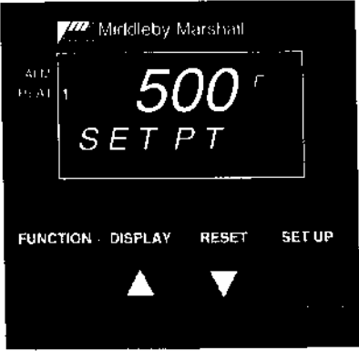
Grey Digital Temperature Controller (Former Style) Contrôleur numérique gris de température (Ancien modèle)
