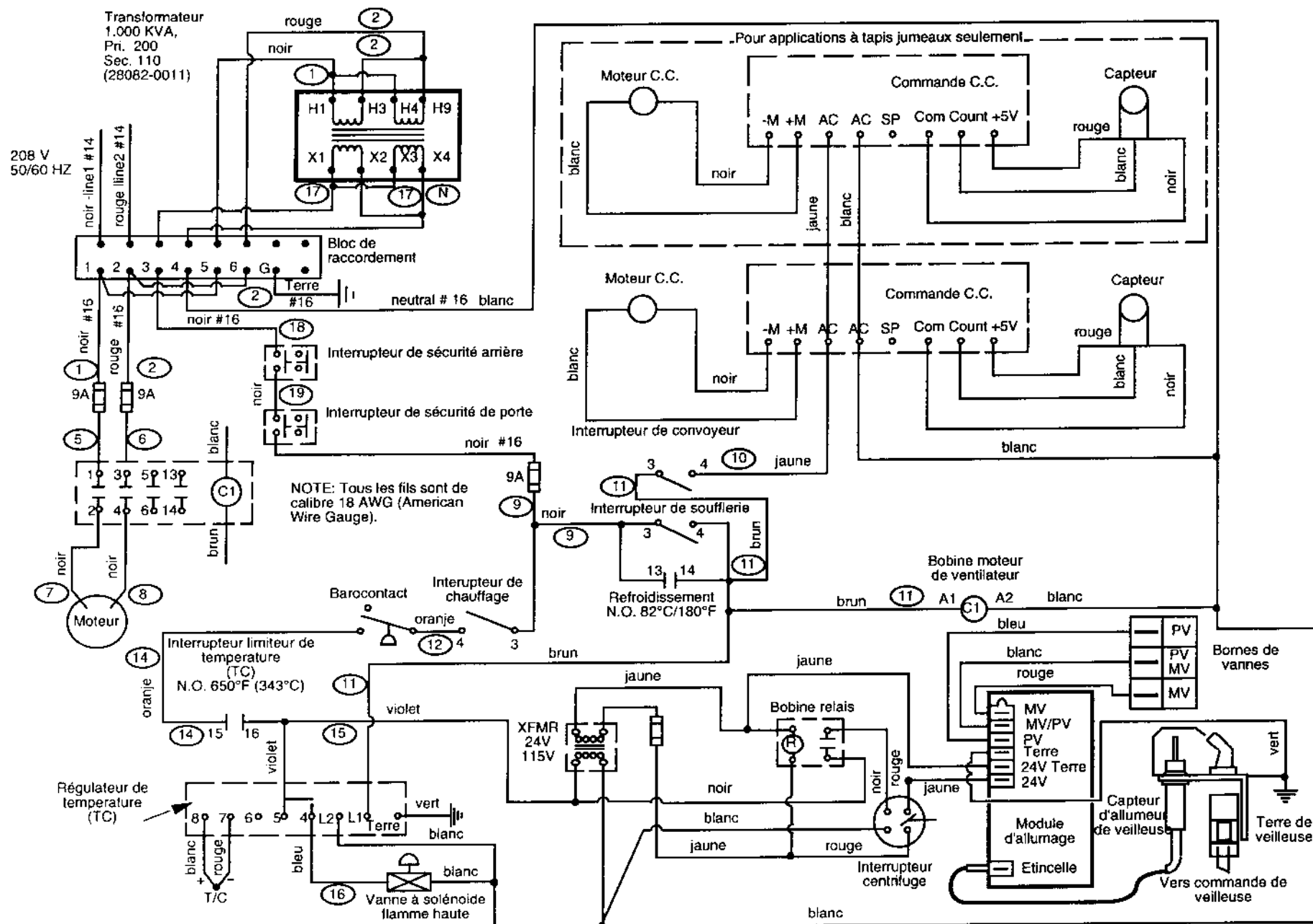
SCHEMA DE CÂBLAGE DU FOUR À GAZ SÉRIE PS200 Moteur de soufflerie 208 V, 50/60Hz, 4.,1 A, bipolaire, 3 fils (2 conducteurs, 1 terre), monophasé, Circuit de commande 120V, EXPORTATION SEULEMENT
