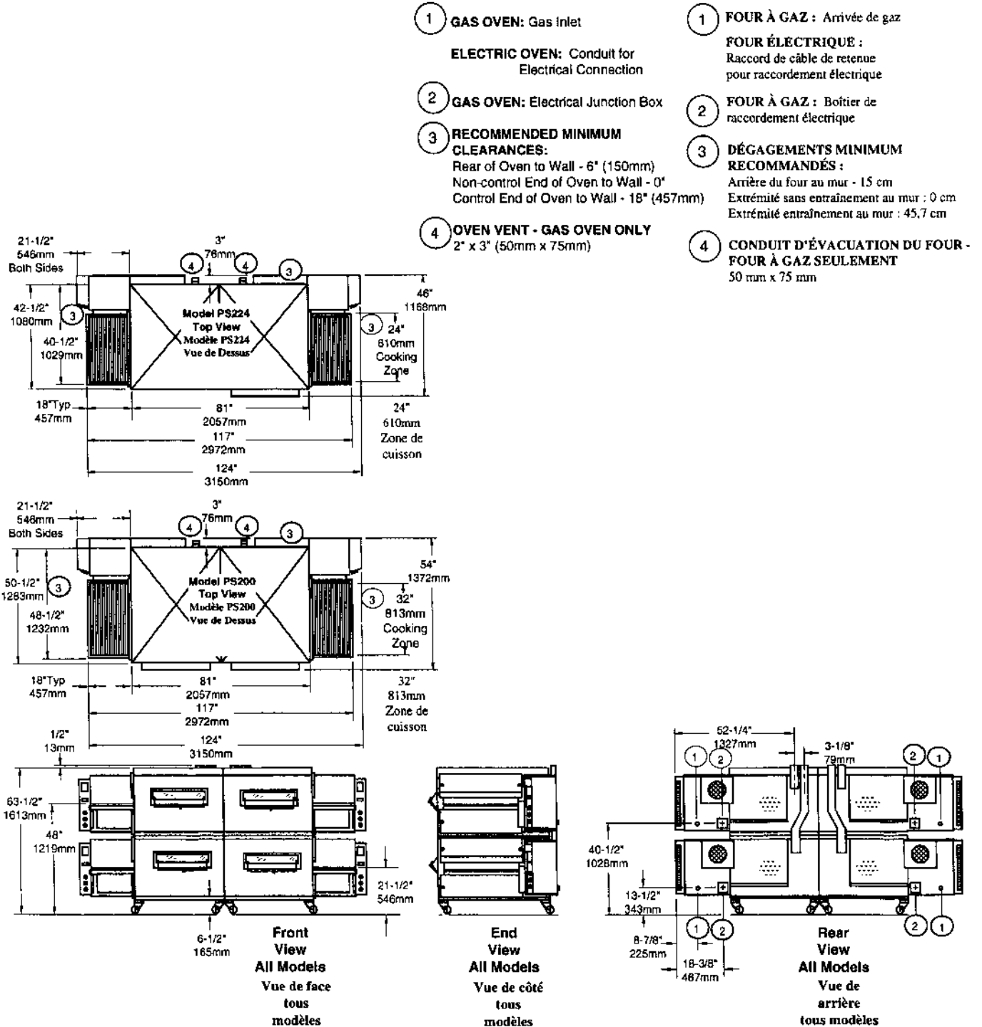
Figure 2-11. MODÈLES PS200 & PS224 FOURS TANDEM DOUBLES MODÈLES PS200 ET PS 224 - DIMENSIONS
