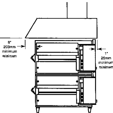
Figure 2-19 Hotte d'aération
