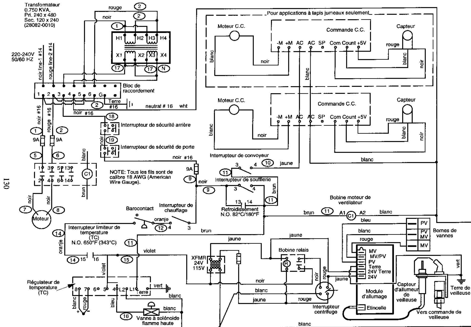
SCHÉMA DE CÂBLAGE DU FOUR À GAZ SÉRIE PS200 Moteur de soufflerie 220-240 V, 50/60Hz, monophasé, 4,1 A, bipolaire, 3 fils (2 conducteurs, 1 terre), Circuit de commande 120V, EXPORTATION SEULEMENT
