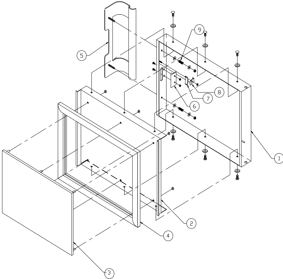
Fig. 5 Door Assembly
