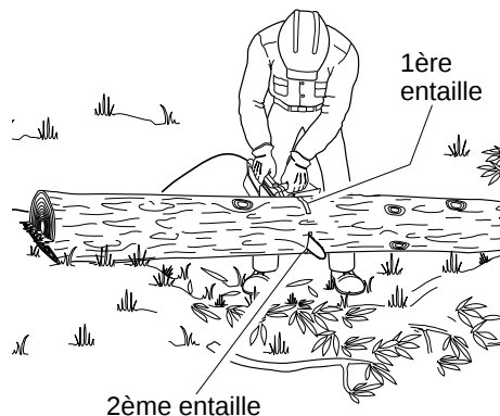
Figure 16 - Tronçonnage d'une bille soutenue aux deux extrémités
