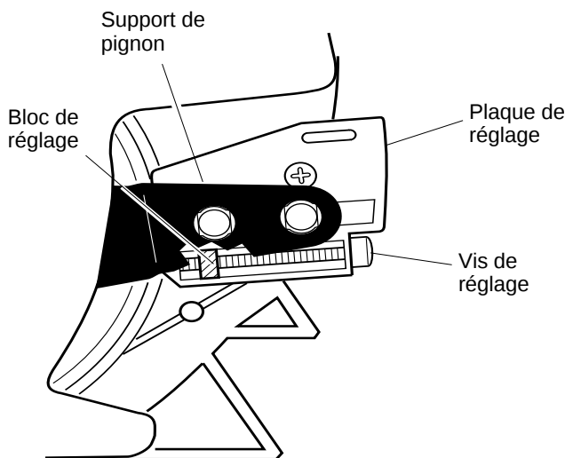
Figure 4 - Emplacement des pièces pour l'assemblage de la lame-guide
