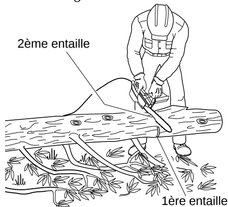
Figure 15 - Tronçonnage d'une bille soutenue à une extrémité
