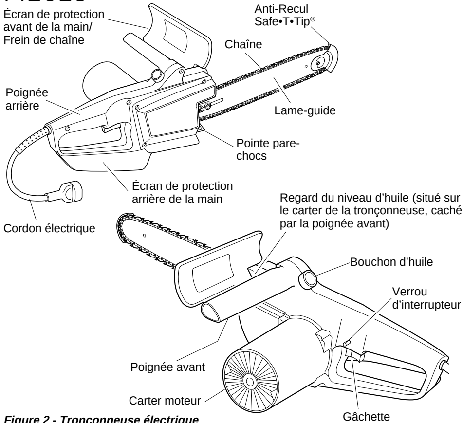
Figure 2 - Tronçonneuse électrique
