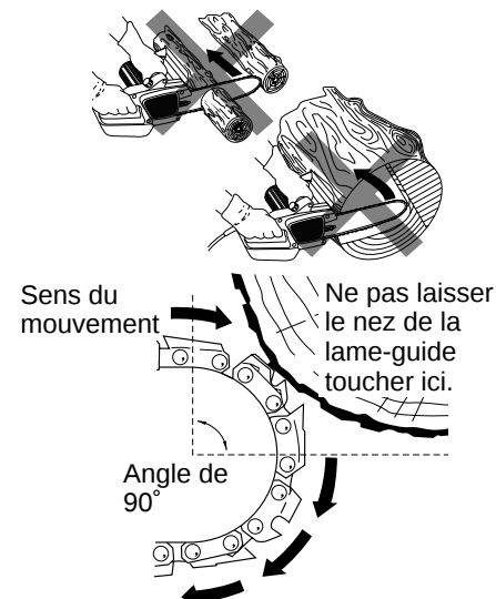
Figure 1 - Exemple du risque de recul. Ne pas laisser le nez de la lame-guide toucher un objet pendant que la chaîne est en mouvement.
