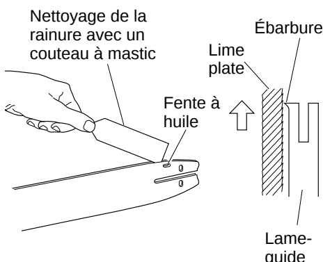
Figure 19 - Entretien de la lame-guide
