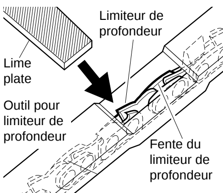
Figure 22 - Position de l'outil pour limiteur de profondeur sur la chaîne
