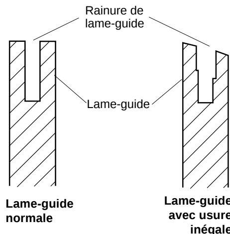
Figure 18 - Coupe transversale d'une lame-guide montrant une usure inégale
