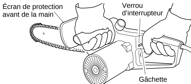
Figure 9 - Emplacement de l'écran de protection avant de la main, du verrou d'interrupteur et de la gâchette
