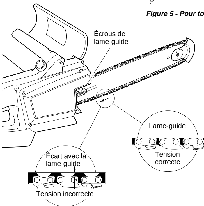
Figure 6 - Réglage de la chaîne
