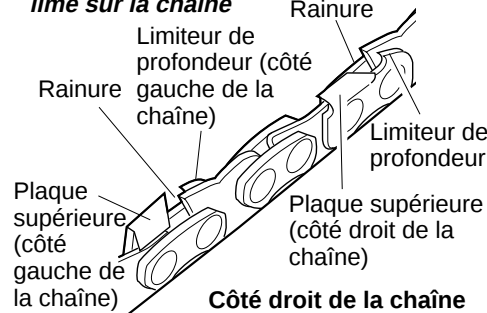
Figure 21 - Emplacement des pièces de la chaîne
