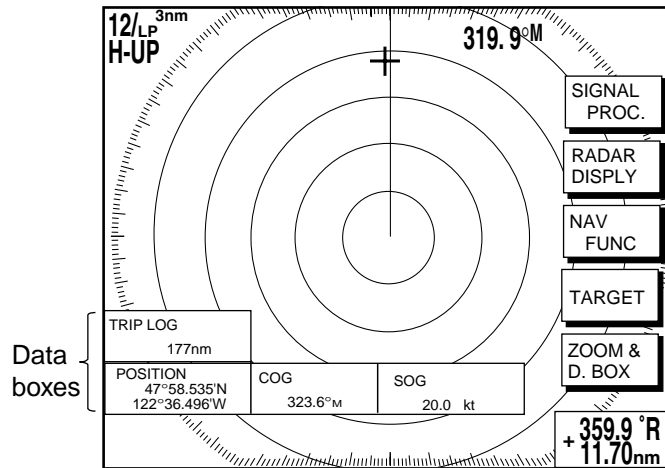
Radar Display
